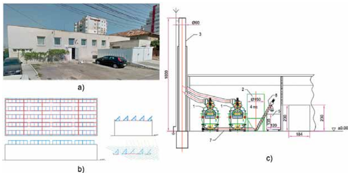
Figura nr. 5. Soluția de conversie a unui punct termic a) într-o centrală cu surse regenerabile incluzând panouri solare termice b) și două centrale termice cu peleți c)
