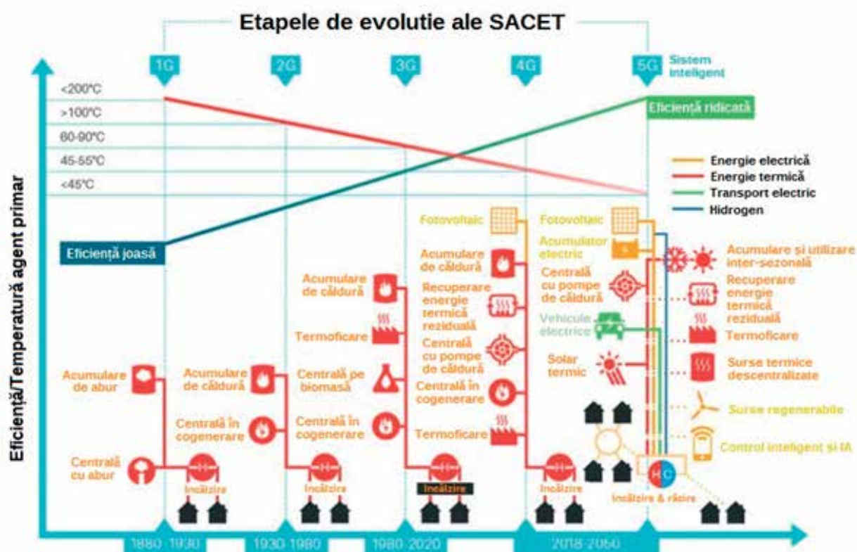
Figura nr. 3. Stadiile de evoluție tehnologică ale SACET pe plan modal
